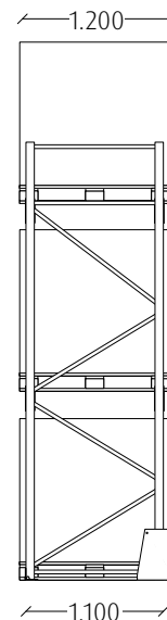
Seitenansicht
